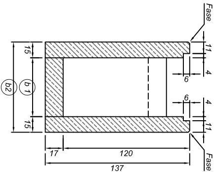
SCHNITT B-B
