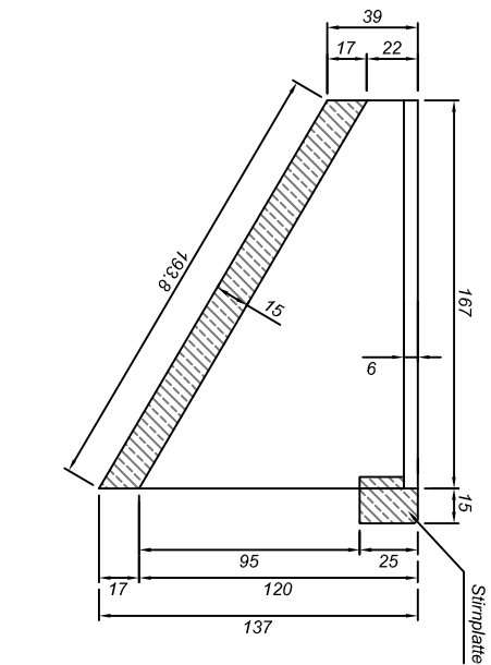
SCHNITT A-A
